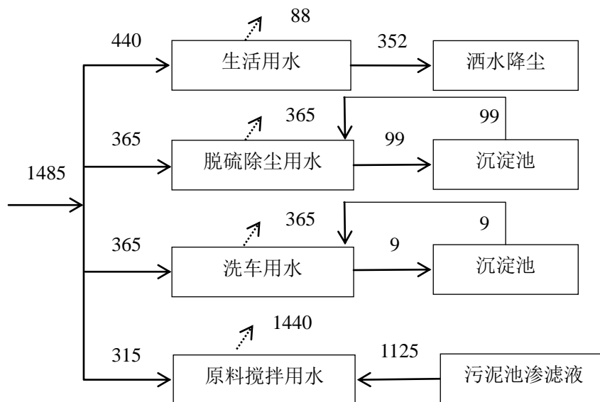
图 2.2.5.2-1 厂水平衡图 (m 3 /a)
