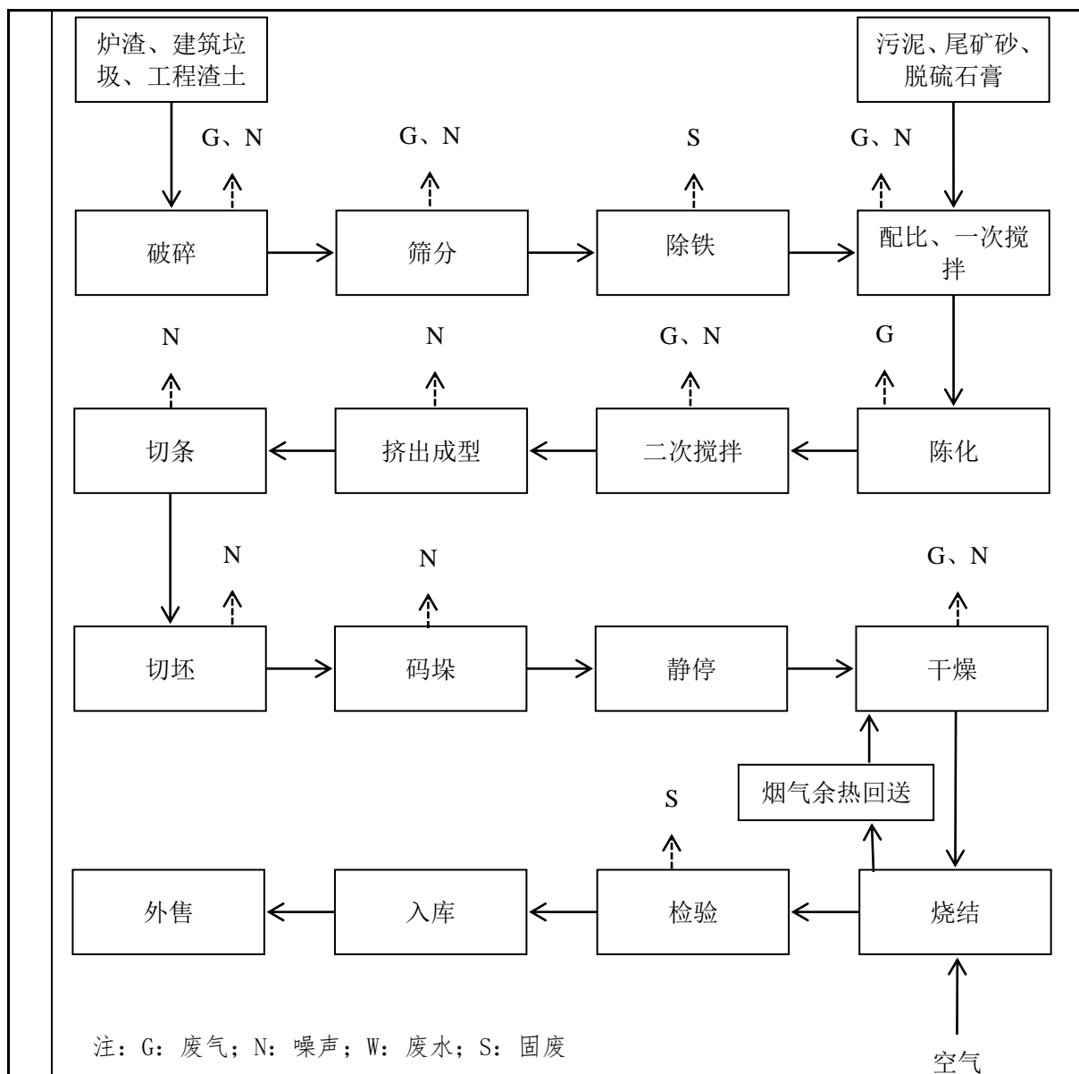
图 2.4-1 运营期工艺流程及产排污节点图
