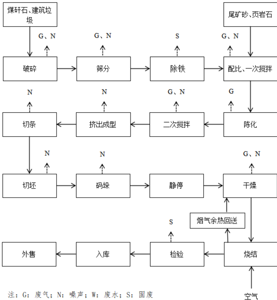
图 2.1.6-1 工艺流程及排污节点图
