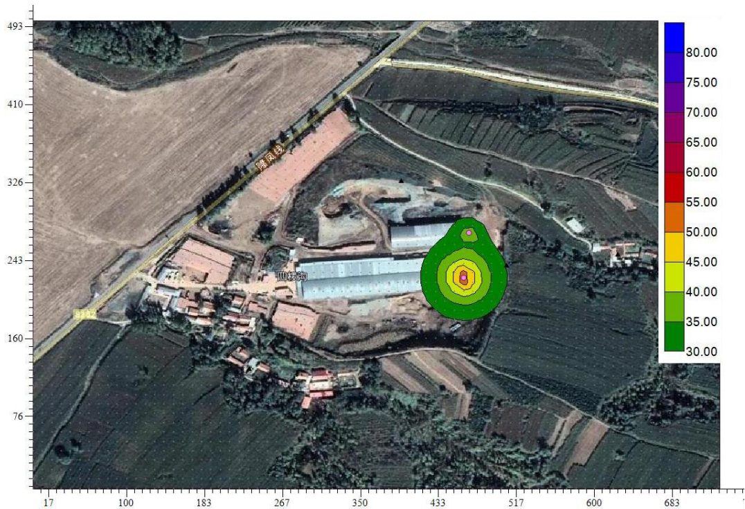
图 4.2.3.3-1 噪声贡献值等声级线图
