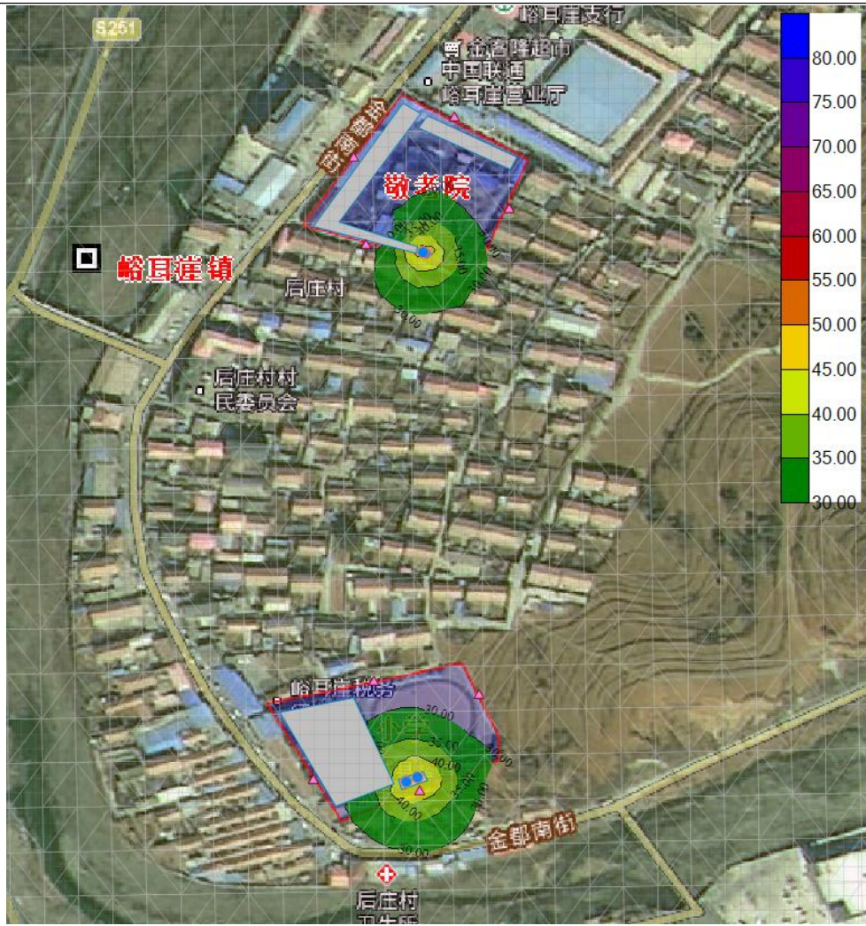
图 4-1 峪耳崖小学和敬老院噪声等值线图
