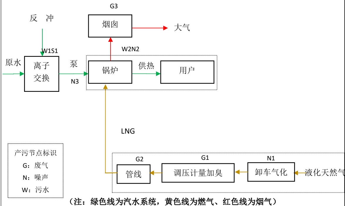
图 2-1 锅炉、LNG 加压站工艺流程图
