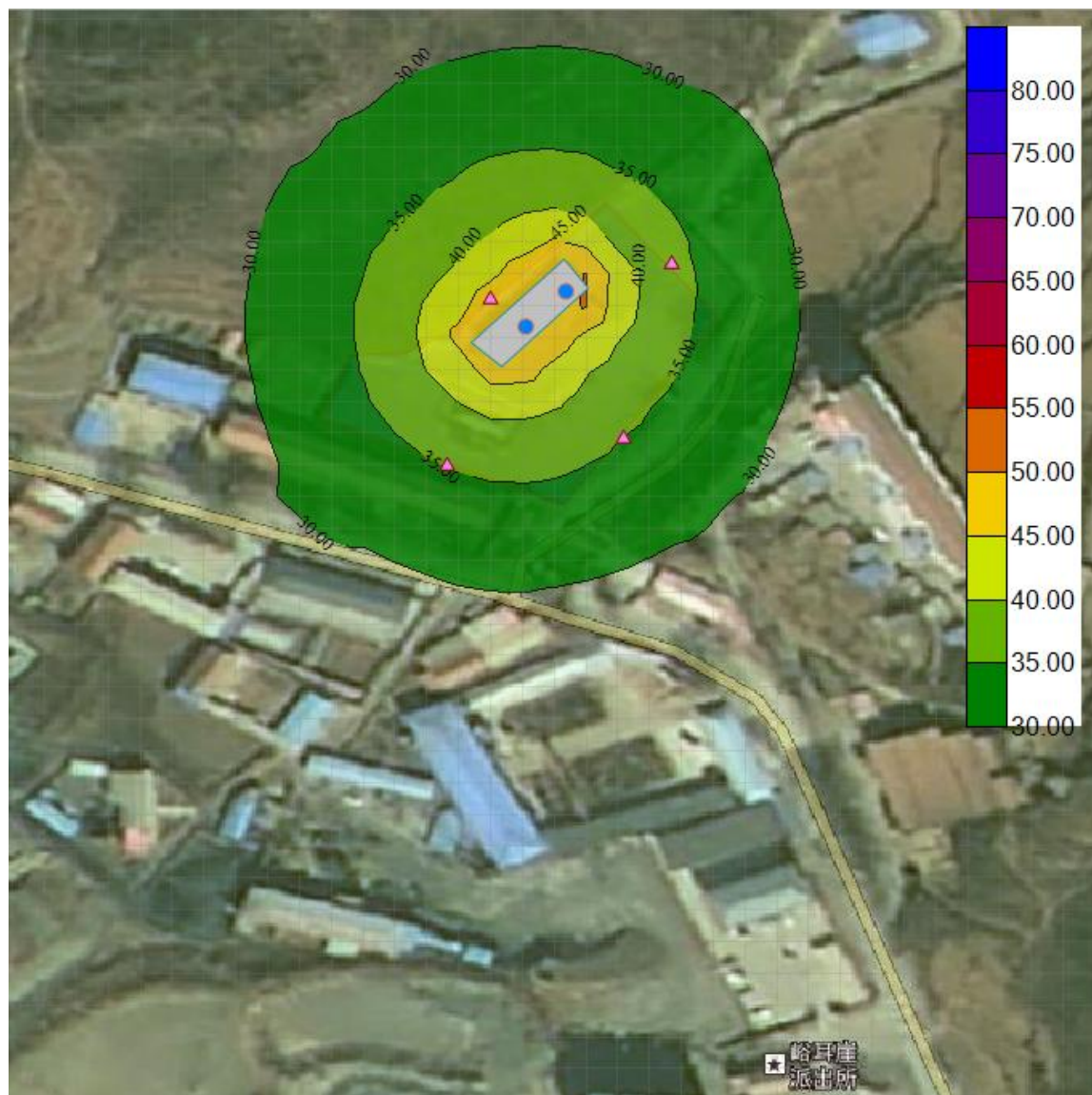
图 4-3 峪耳崖镇加气站噪声等值线图 噪声源监测方案详见下表：
