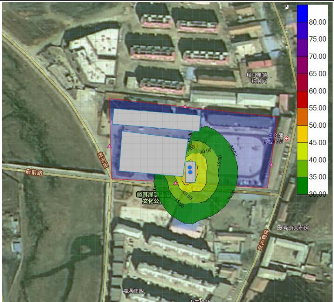
图 4-2 峪耳崖镇政府噪声等值线图
