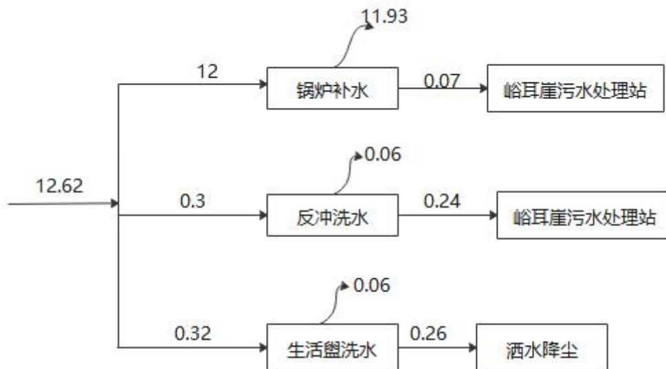
图 1-1 水平衡图 ( \text{m}^3/\text{d} )
